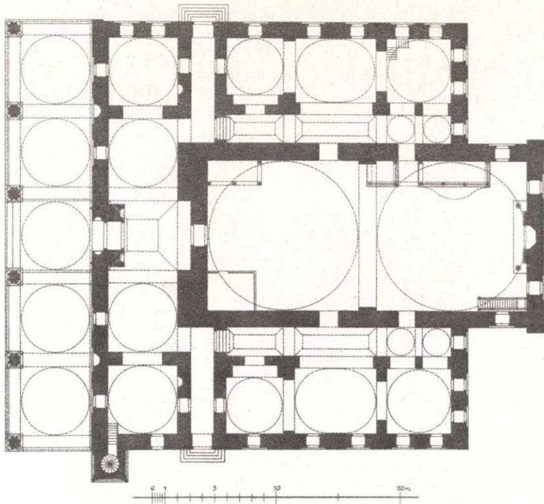
15,a MOSCHEE DES MAHMUD PASCHA, GRUNDRISS
