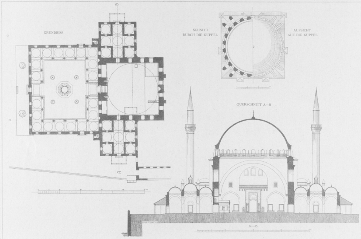
17,b MOSCHEE DES SULTAN SELIM I. (SELIMIE)
